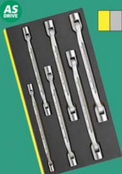
6 scharniersleutels, 8x9, 10x11, 12x13, 14x15, 16x17 en 18x19 mm
